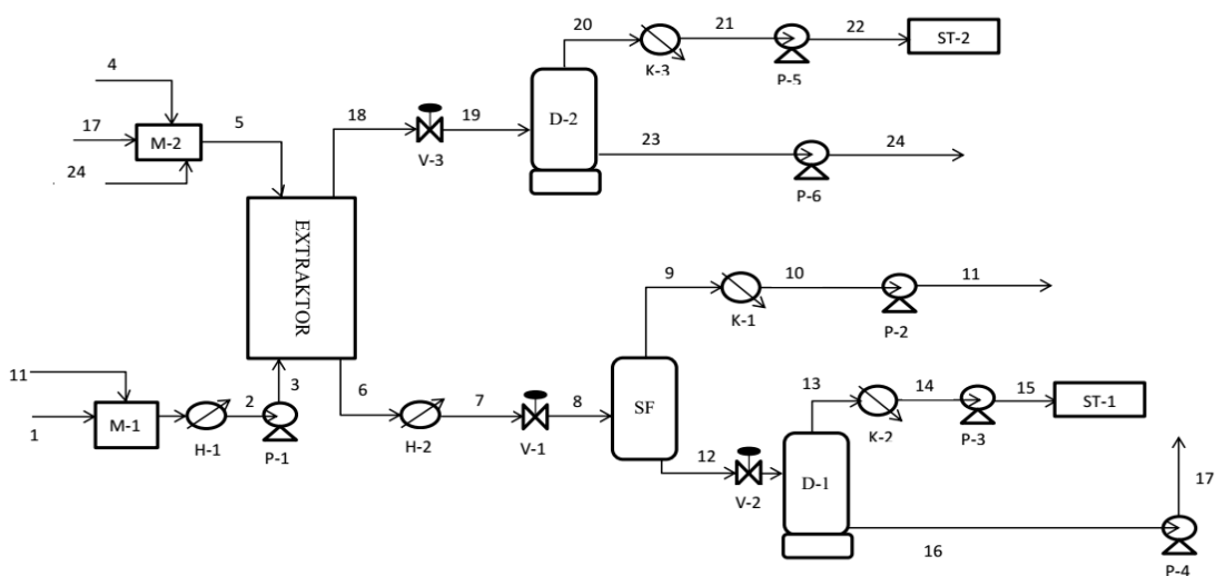
Obr. 1 Prúdová schéma navrhutého procesu: H-1, H-2 – ohrievač; D-1, D-2 – odparka; V-1, V-2, V-3 – škrtiaci ventil; SF – separátor fáz; P-1, P-2, P-3, P-4, P-5, P-6 – čerpadlo; K-1, K-2, K-3 – kondenzátor; M-1, M-2 – miešač. Prúdy: 1 – surovina; 2 a 3 – ohriata surovina na vstupe do extraktora; 4 – čerstvá IL; 5 – regenerovaná IL na vstupe do extraktora; 6 – finálny extrakt; 7 – ohriaty extrakt; 8 – paro-kvapalná zmes po redukcii tlaku na 50 kPa; 9, 10, 11 – skondenzované pary MTBE a metanolu recirkulované do miešača M-1; 12 – kvapalný zvyšok zo separátora fáz na vstupe do odparky D-1; 13, 14, 15 – prúd produktu metanol; 16, 17 – regenerovaná IL s čistotou 98 mól.% privádzaná do miešača IL M-2; 18 – rafinát z extraktora; 19 – paro-kvapalná zmes rafinátu po redukcii tlaku na 73,5 kPa; 20, 21, 22 – prúd produktu MTBE; 23, 24 – zvyšok s obsahom 25 mól.% IL sa vracia do miešača IL M-2.
